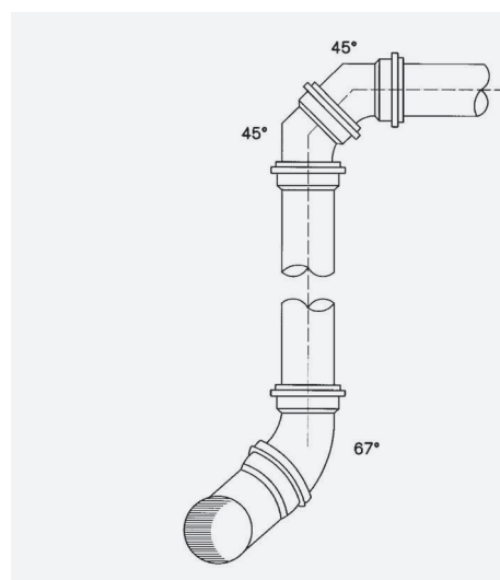
РИС. 12. ПРИМЕР ВЕРТИКАЛЬНОГО ПОДКЛЮЧЕНИЯ К ГЛАВНОМУ КАНАЛИЗАЦИОННОМУ КАНАЛУ
