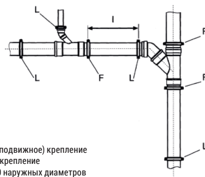
ХОМУТ С ПРОКЛАДКОЙ КАК ПЛАВУЩЕЕ КРЕПЛЕНИЕ
