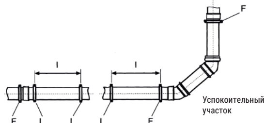
ПРИМЕРЫ РАСПОЛОЖЕНИЯ ЖЕСТКИХ И ПЛАВУЩИХ КРЕПЛЕНИЙ
